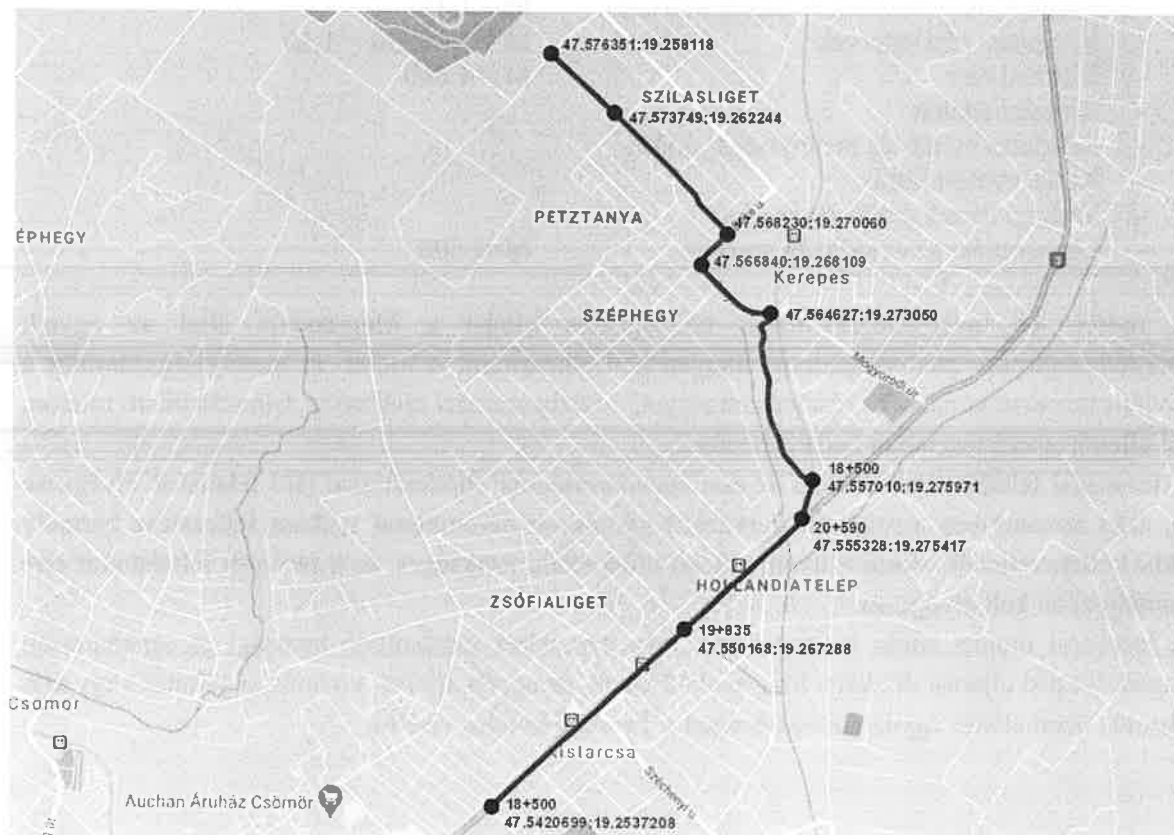
Átnézeti helyszínrajz
